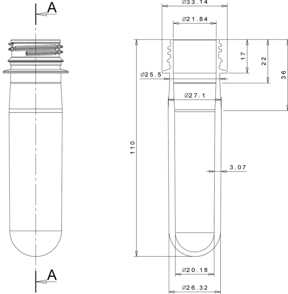
A-A View/Görünüm
